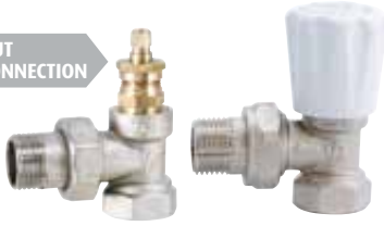
CORNER RADIATOR VALVE Угловой Кран Радиатора. شیر رادیاتور(زانویی)
