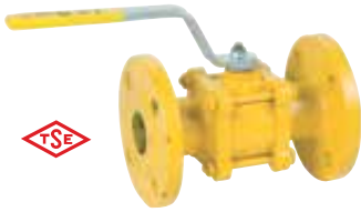
NATURAL GAS BALL VALVE CASTING (PN 40-GGG40-TS EN 331-MOP5) Кран Шаровой для Газа (чугун) (PN 40-GGG40-TS EN 331-MOP5)
