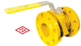
NATURAL GAS BALL VALVE CASTING (PN 16-GGG40-TS 9809-MOP5-TYPE2) Кран Шаровой для Газа (чугун) (PN 16-GGG40-TS 9809-MOP5-TIP2)
